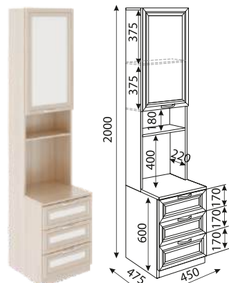
M10 Стеллаж для принтера
