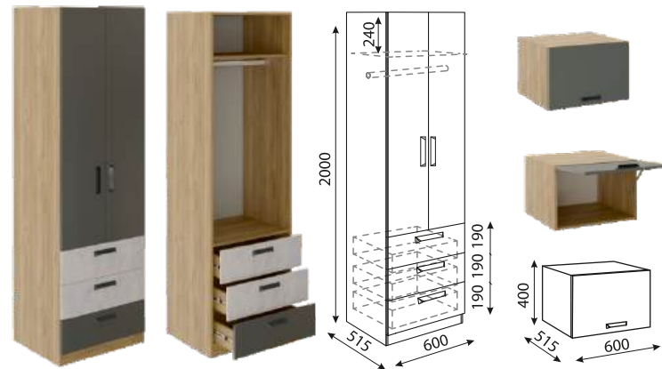
М04 Шкаф с ящиками
