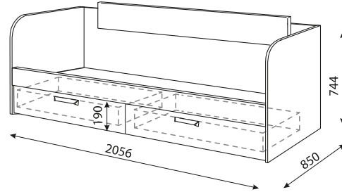
M13 Кровать с ящиками (спальное место 800x2000)
